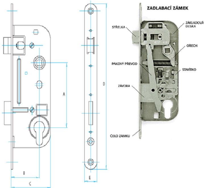
Vložkový zadlabací zámek s převodem
