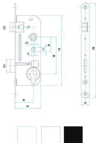
Vložkový zadlabací zámek s převodem
