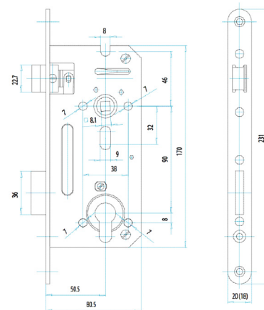
Vložkový zadlabací zámek s převodem
